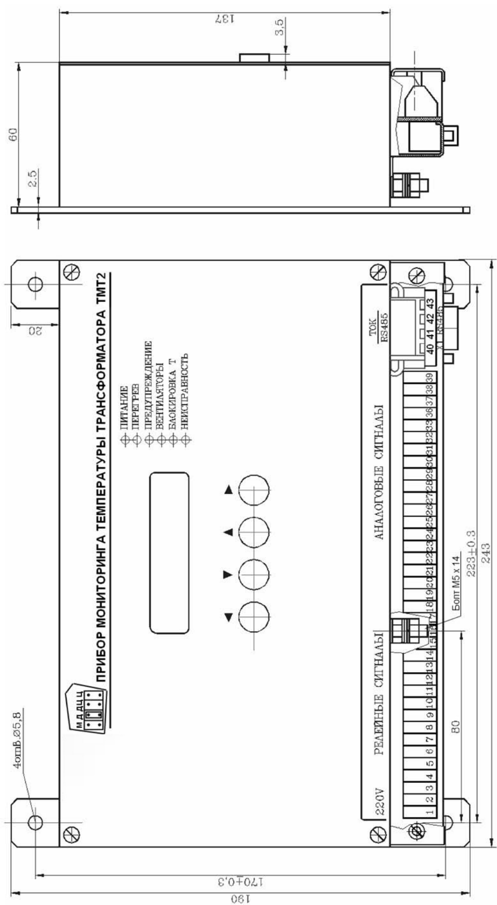
Габаритный чертёж приборов
